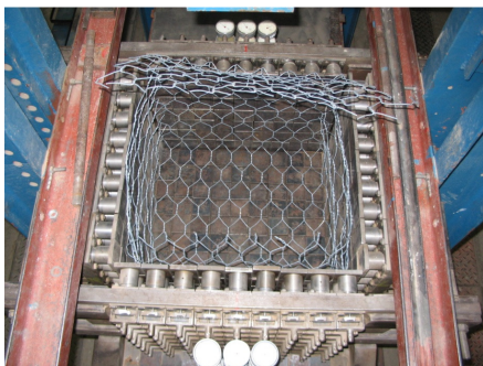
Rys. 2. Widok z góry na wnętrzu pojemnika badawczego, w którym umieszczono model fizyczny kosza siatkowego z kruszywem (gabionu) [5, 7] Fig. 2. Top view of the interior of the container research, which indicates a physical model of aggregate mesh basket (gabion) [5, 7]
