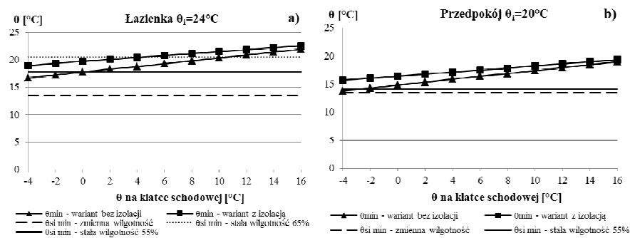
Rys. 5. Porównanie \theta_{min} z \theta_{simin} : a) łazienka, b) przedpokój
