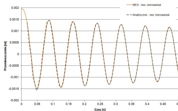
Rys. 3. Przeszyczenie końca belki w drganiach swobodnych liczone metodą analityczną oraz MES
