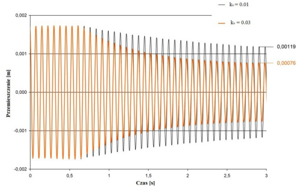
Rys. 6. Przeszyczenie końca belki przy różnych współczynnikach wzmacnienia – model bez warstwy kleju
