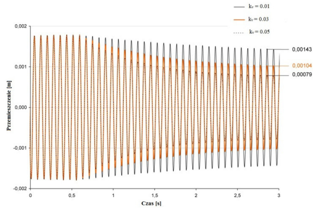
Rys. 7. Przeszyczenie końca belki przy różnych współczynnikach wzmacnienia – model z warstwą kleju
