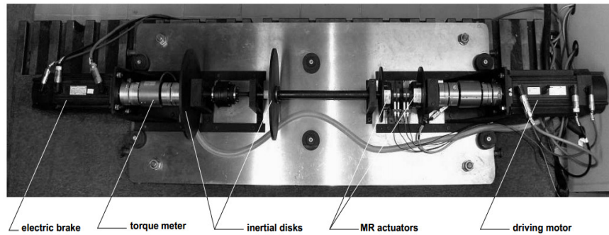
Rys. 1. Stanowisko laboratoryjne
