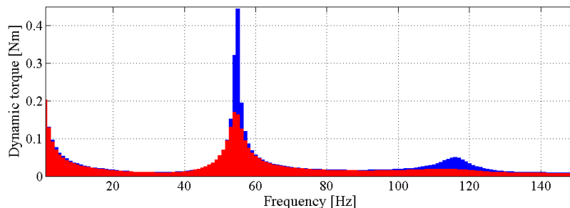
Rys. 3. Obliczone amplitudowe charakterystyki momentu dynamicznego (układ niethumiony- kolor niebieski, układ tłumiony- kolor czerwony)
