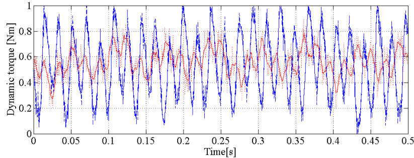
Rys. 4. Zmierzony przebieg momentu dynamicznego (układ nietyumiony- kolor niebieski, układ tłumiony- kolor czerwony)
