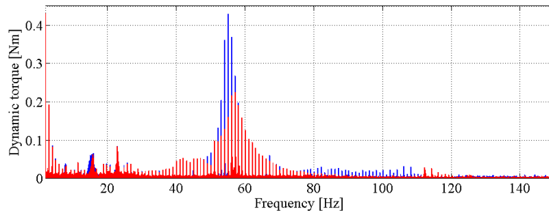
Rys. 5. Amplitudowe charakterystyki momentu dynamicznego zmierzone doświadczenie (układ nietyumiony- kolor niebieski, układ tłumiony- kolor czerwony)
