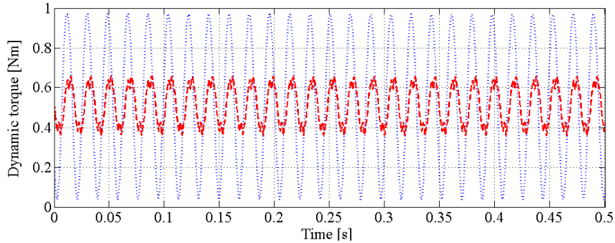
Rys. 2. Obliczony przebieg momentu dynamicznego (układ niethumiony- kolor niebieski, układ tłumiony- kolor czerwony)
